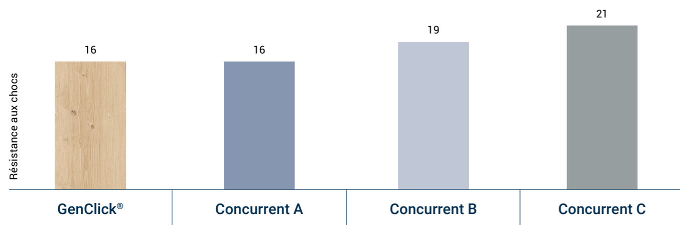
GRAPHIQUE 2 : RÉSISTANCE AUX CHOCS (TEST INTERNE)
