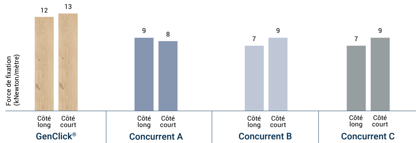
GRAPHIQUE 1 : FORCE DE FIXATION (ISO 10582) UN SCORE ÉLEVÉ DE LA FORCE DE FIXATION = UN ASSEMBLAGE PLUS SOLIDE
