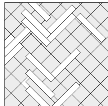
Verlegemuster
